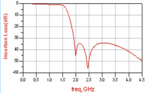
● LFCN3216-1325A01
